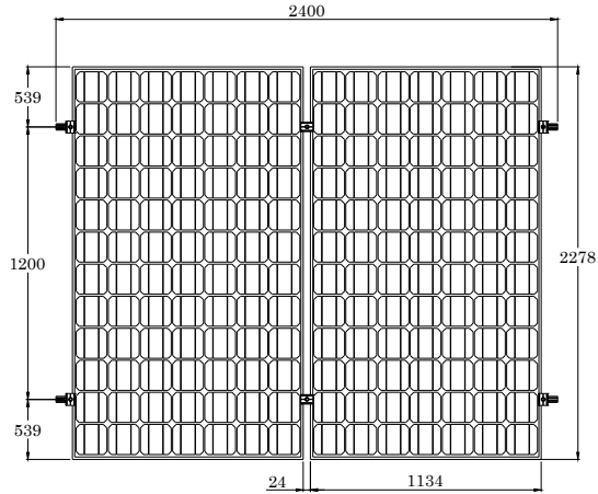
VISTA PLANTA
