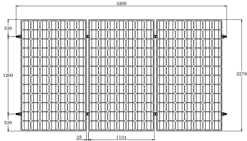
VISTA PLANTA
