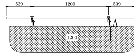
VISTA LATERAL
